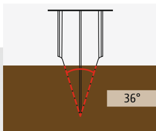
Ciężka gleba Podparcie na profilu pierścienia
