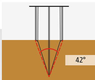
Lekka gleba Podparcie na grzbiecie pierścienia
