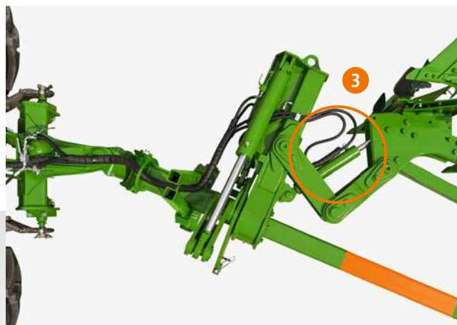
Hydrauliczna regulacja pierwszego korpusu
